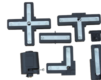
레일연결 부속
