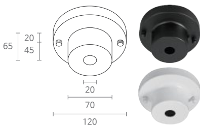
Color : black, white 전선홀 : Ø20 Size (Circle uneven) W120 x D120 x H25(70 x 70 x 40) mm
