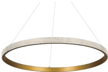
트라이(대) 1단 80W P/D Size : Ø800 x H40 mm Color : Gold Color temperature : 4000K (오스람칩/KS제품) OSRAM
