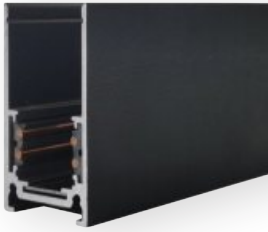
마그네틱 트랙 A타입 Color : black / Width : 1m, 2m, 3m Size : W27 x 52 mm / 타공사이즈 : 29 mm Type : 직부, 매입, 펜던트 가능 직렬 최대 10m 이하 사용
