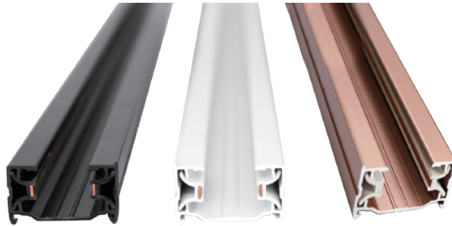
블랙 (절연체 / 프레임 색 동일) 화이트 (절연체 / 프레임 색 동일) 로즈골드 (절연체 흰색 / 프레임 로즈골드)
